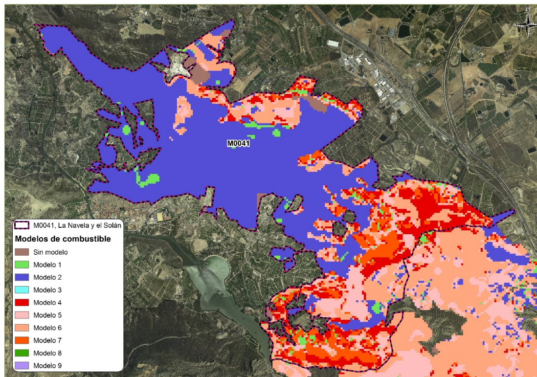
FIGURA 22. Modelos de combustible
