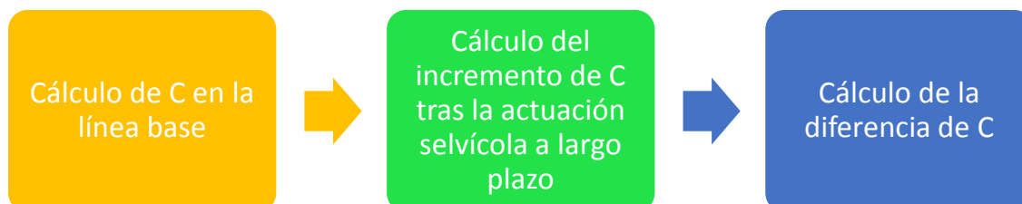
FIGURA 48. Procedimiento para el cálculo del sumidero de carbono
