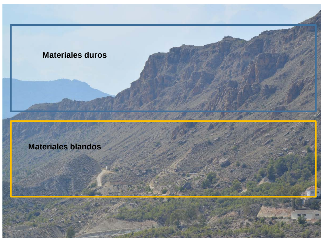
FIGURA 26. Disposición de los materiales de ladera en el MUP - 41
