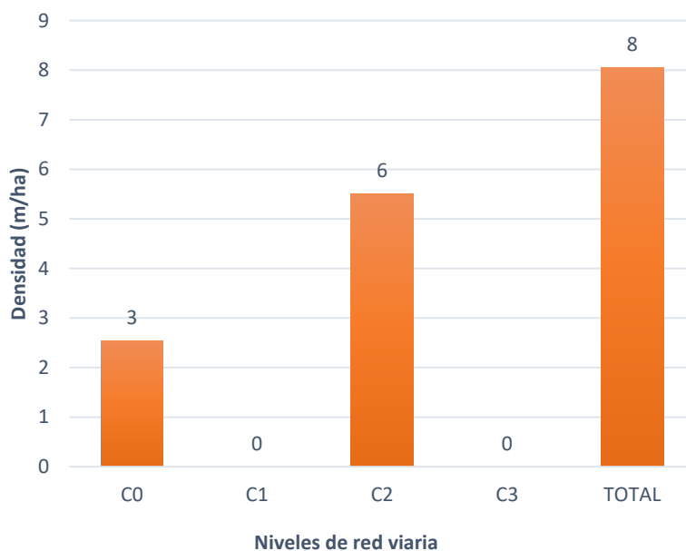
FIGURA 30. Análisis de la densidad de red viaria clasificada por órdenes o niveles
