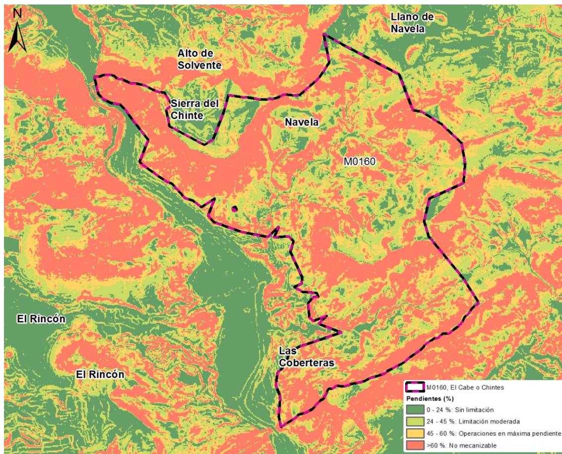
FIGURA 32. Limitaciones por pendientes
