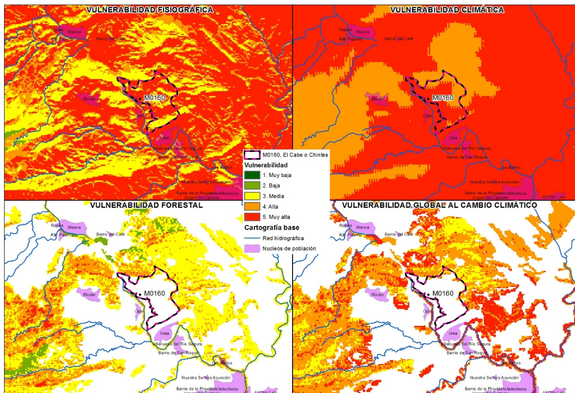
FIGURA 16. Análisis de vulnerabilidades frente al cambio climático
