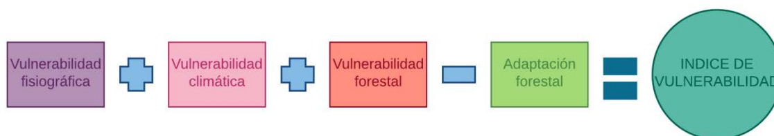
FIGURA 15. Vulnerabilidad global frente al cambio climático
