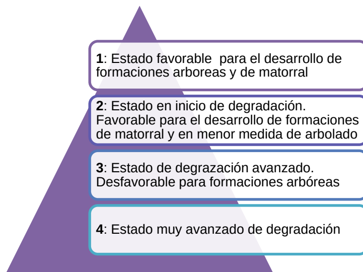
FIGURA 40. Calidades de estación
