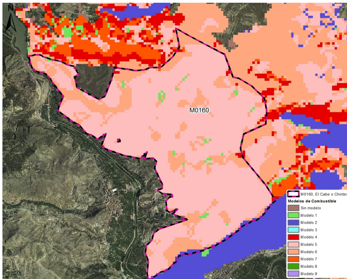
FIGURA 22. Modelos de combustible
