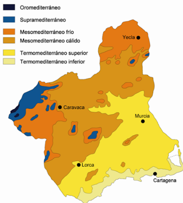
FIGURA 39. Termotipos para la región de Murcia
