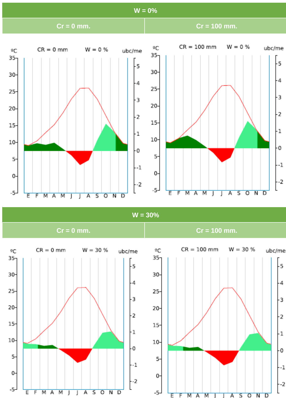
FIGURA 9. Diagramas bioclimáticos MUP – 160
