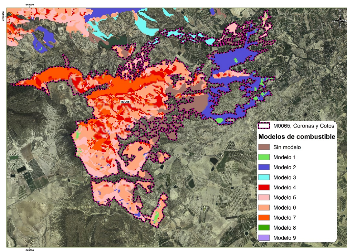
FIGURA 22. Modelos de combustible
