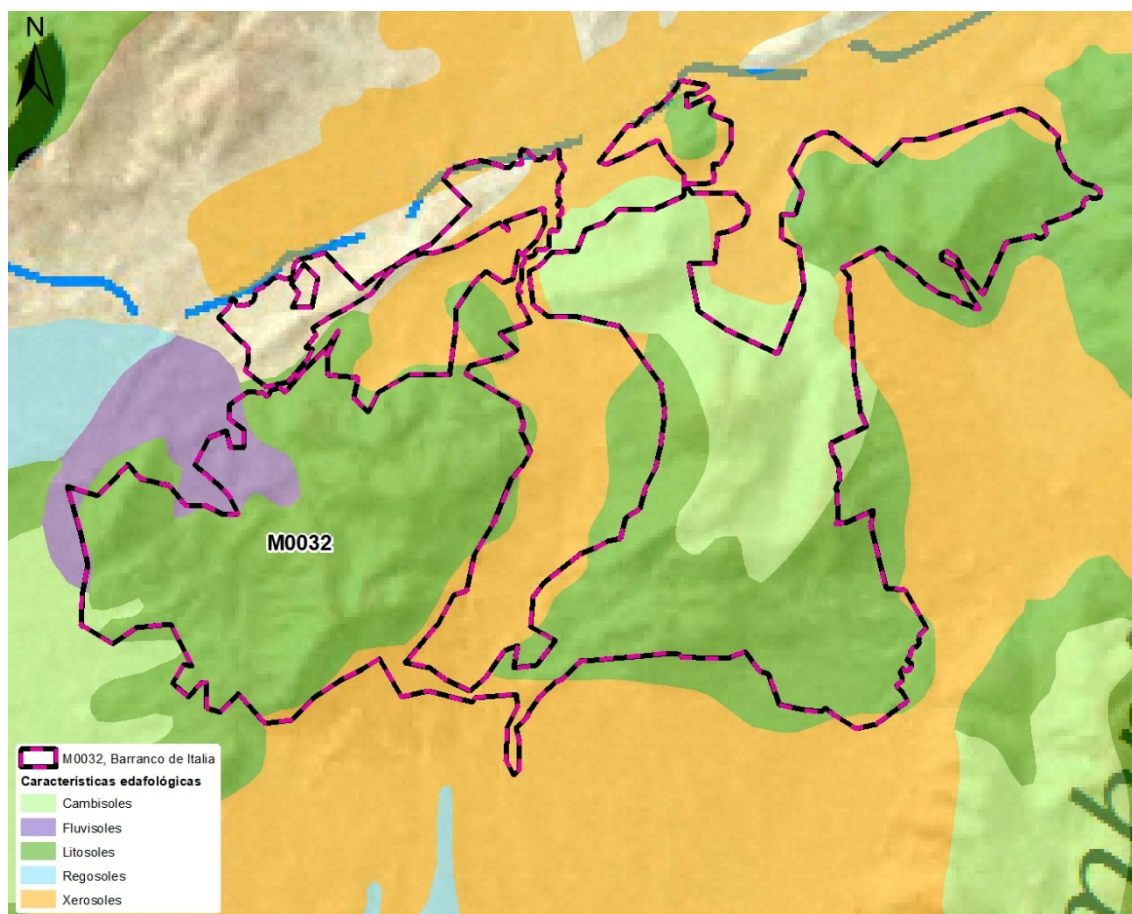
FIGURA 2. Características edafológicas
