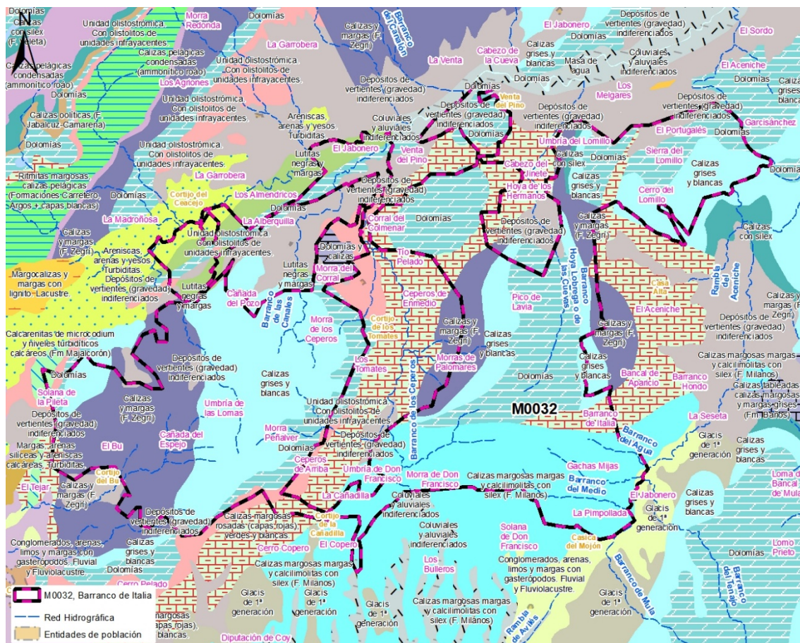
FIGURA 1. Geología
