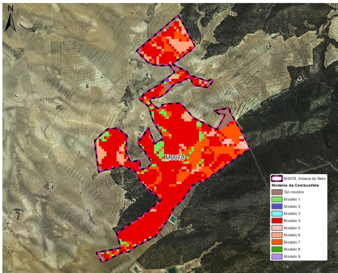
FIGURA 23. Modelos de combustible
