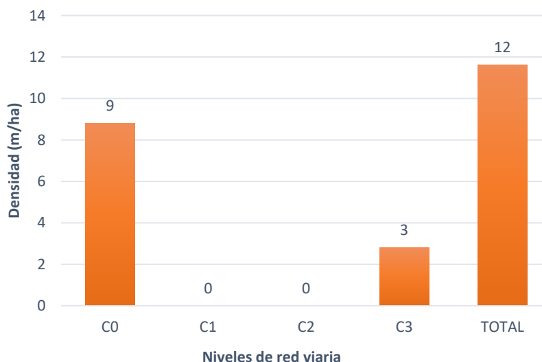
FIGURA 31. Análisis de la densidad de red viaria clasificada por órdenes o niveles
