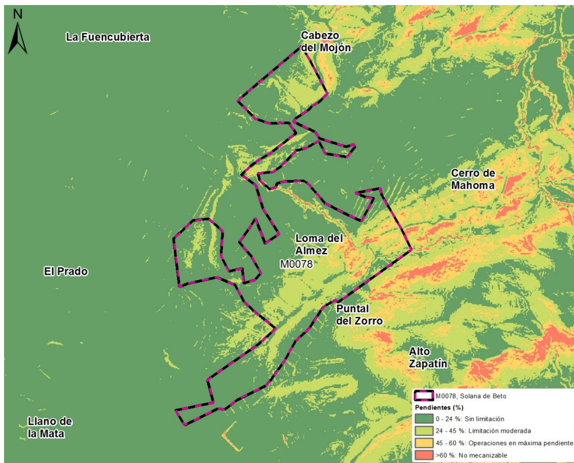
FIGURA 33. Limitaciones por pendientes
