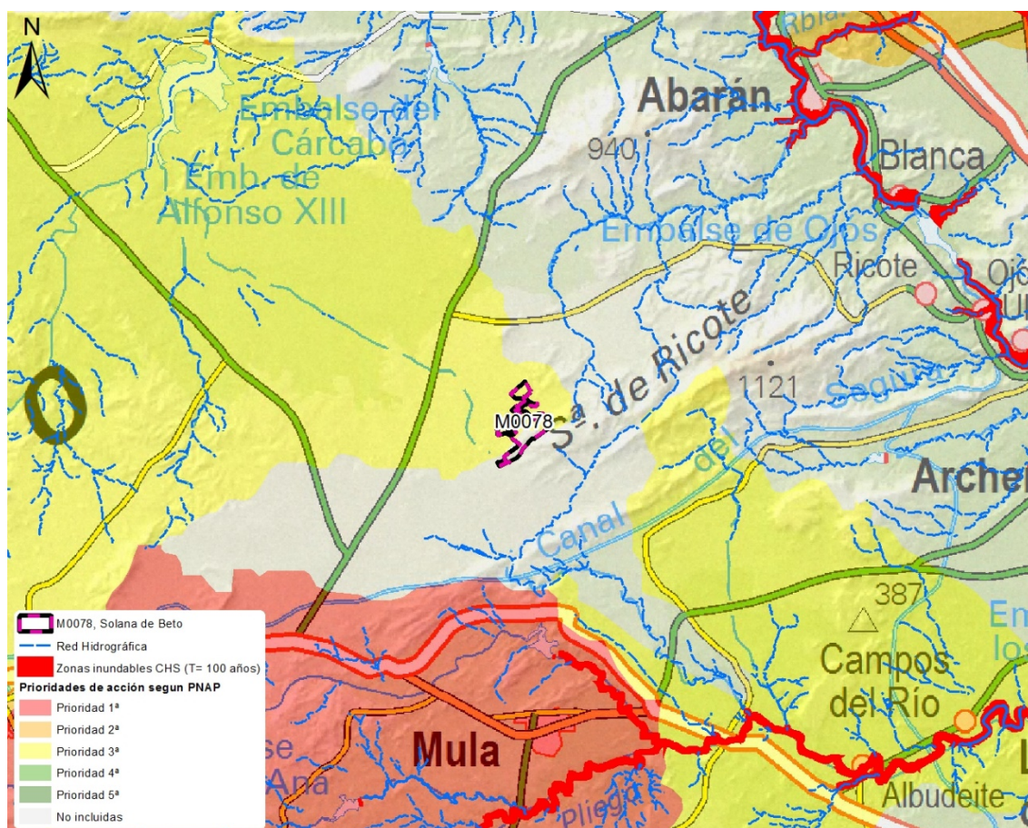
FIGURA 26. Riesgo de inundación
