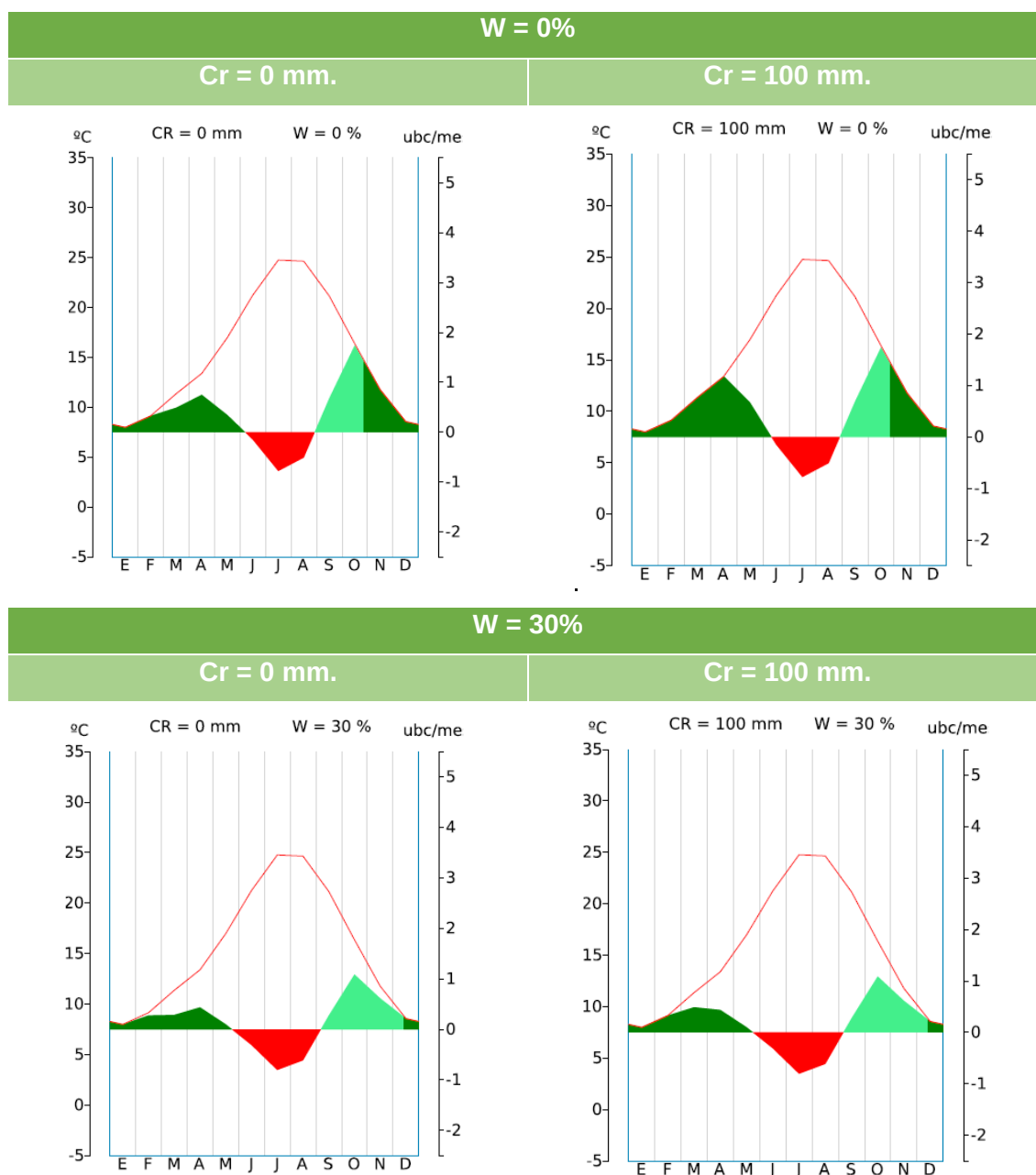
FIGURA 9. Diagramas bioclimáticos MUP – 76
