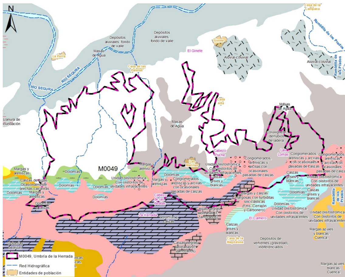
FIGURA 2. Geología
