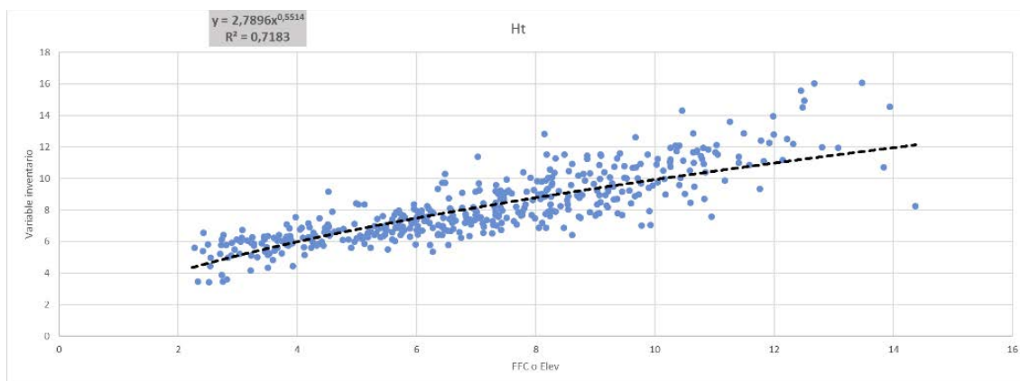
GRÁFICO 3. Gráfica de regresión para la altura total
