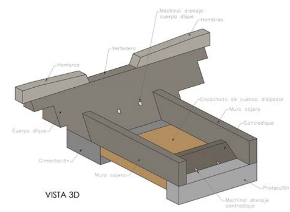
FIGURA 44. Modelo 3D de dique
