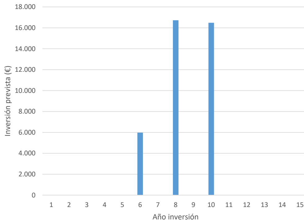
GRÁFICO 6. Inversión en prevención de gestión y mejora de la red viaria por anualidades en el MUP – 44
