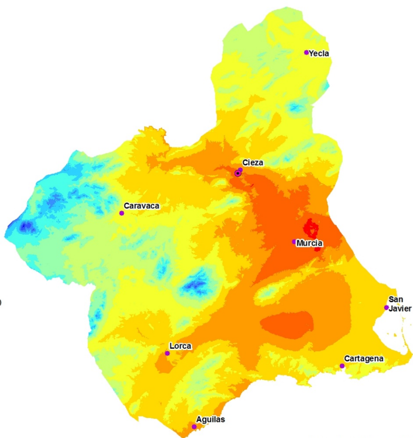
FIGURA 5. T a max anual (°C)
