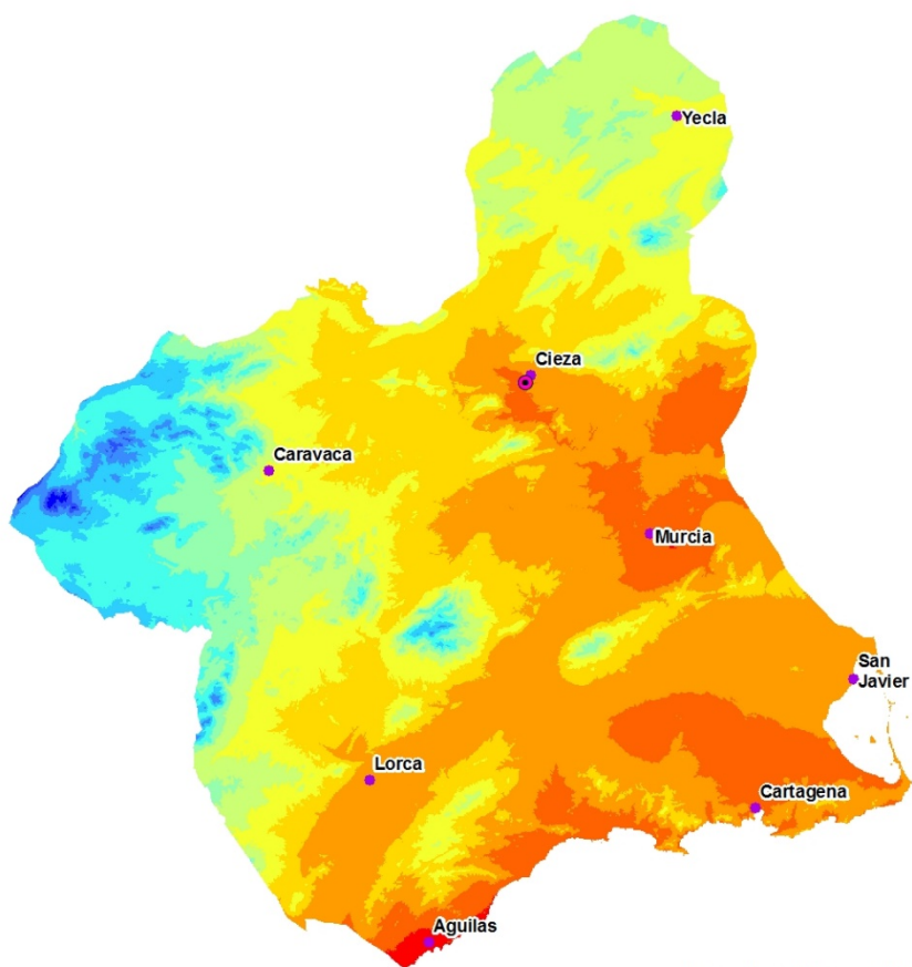
FIGURA 4. Tª media anual (°C)
