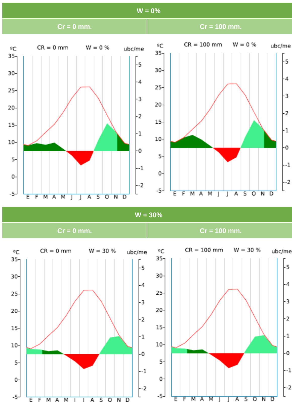
FIGURA 9. Diagramas bioclimáticos MUP – 147
