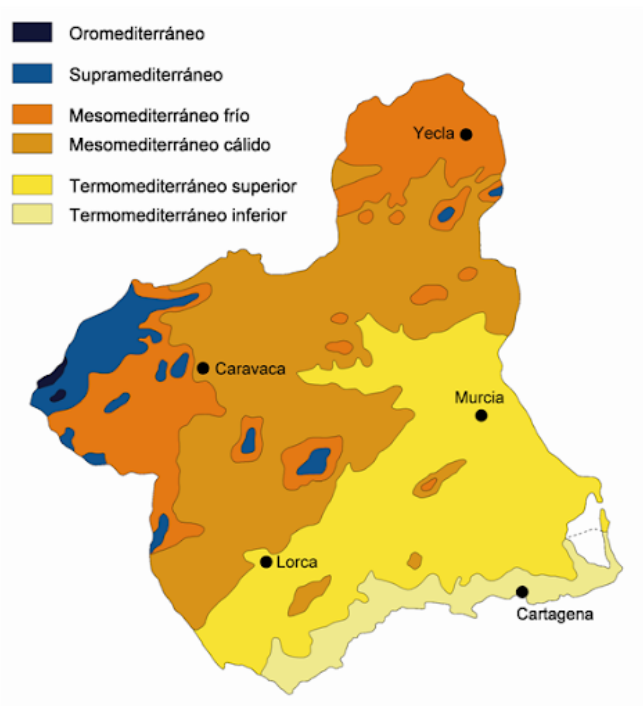
FIGURA 38. Termotípos para la región de Murcia
