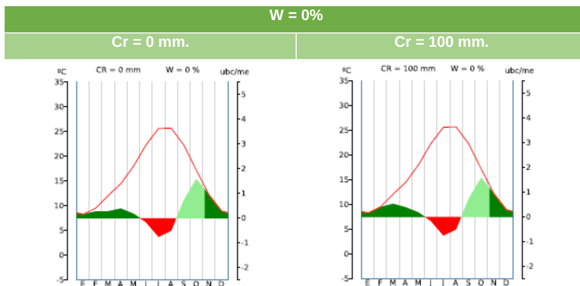
FIGURA 9. Diagramas bioclimáticos
