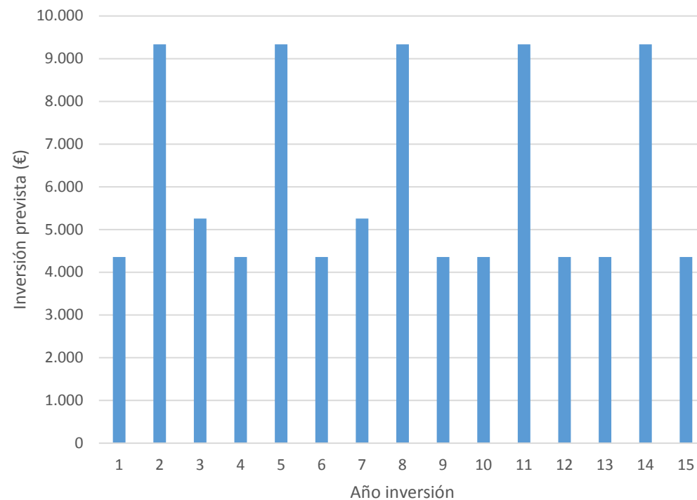
GRÁFICO 4. Inversión en actuaciones de mejora para la fauna por anualidades en el MUP – 139
