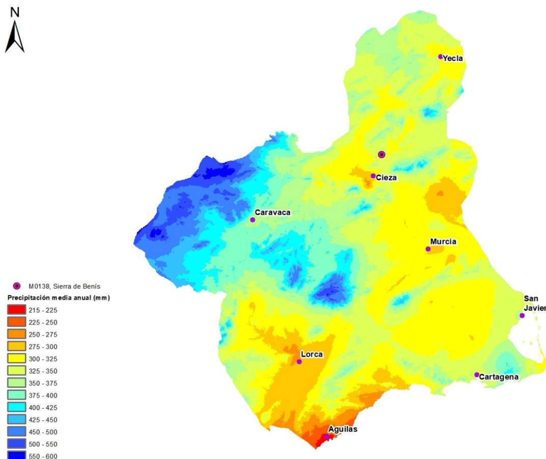
FIGURA 7. Precipitación media (mm)
