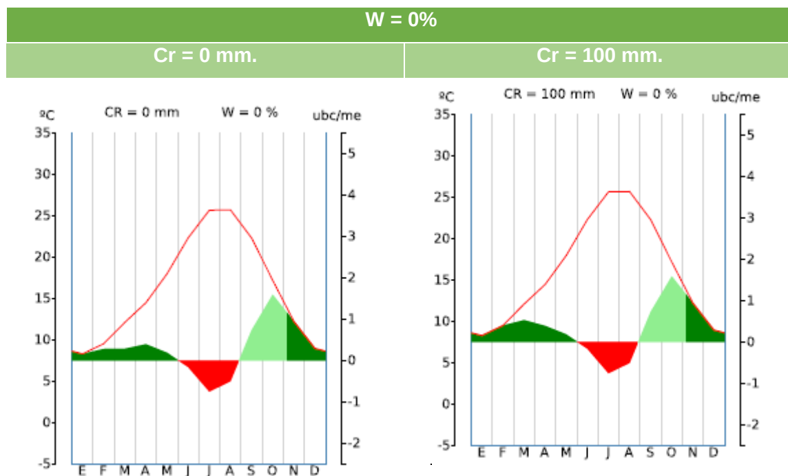
FIGURA 9. Diagramas bioclimáticos
