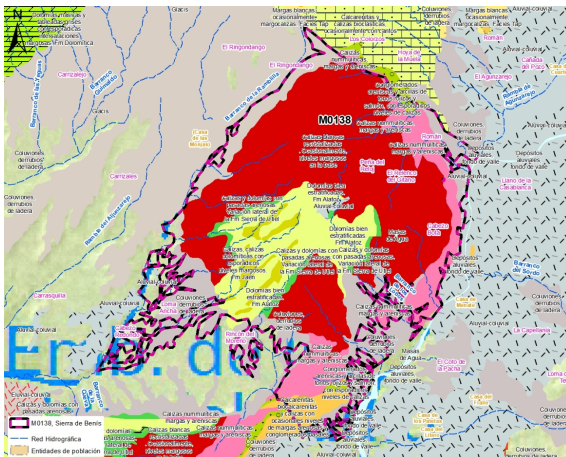
FIGURA 2. Geología
