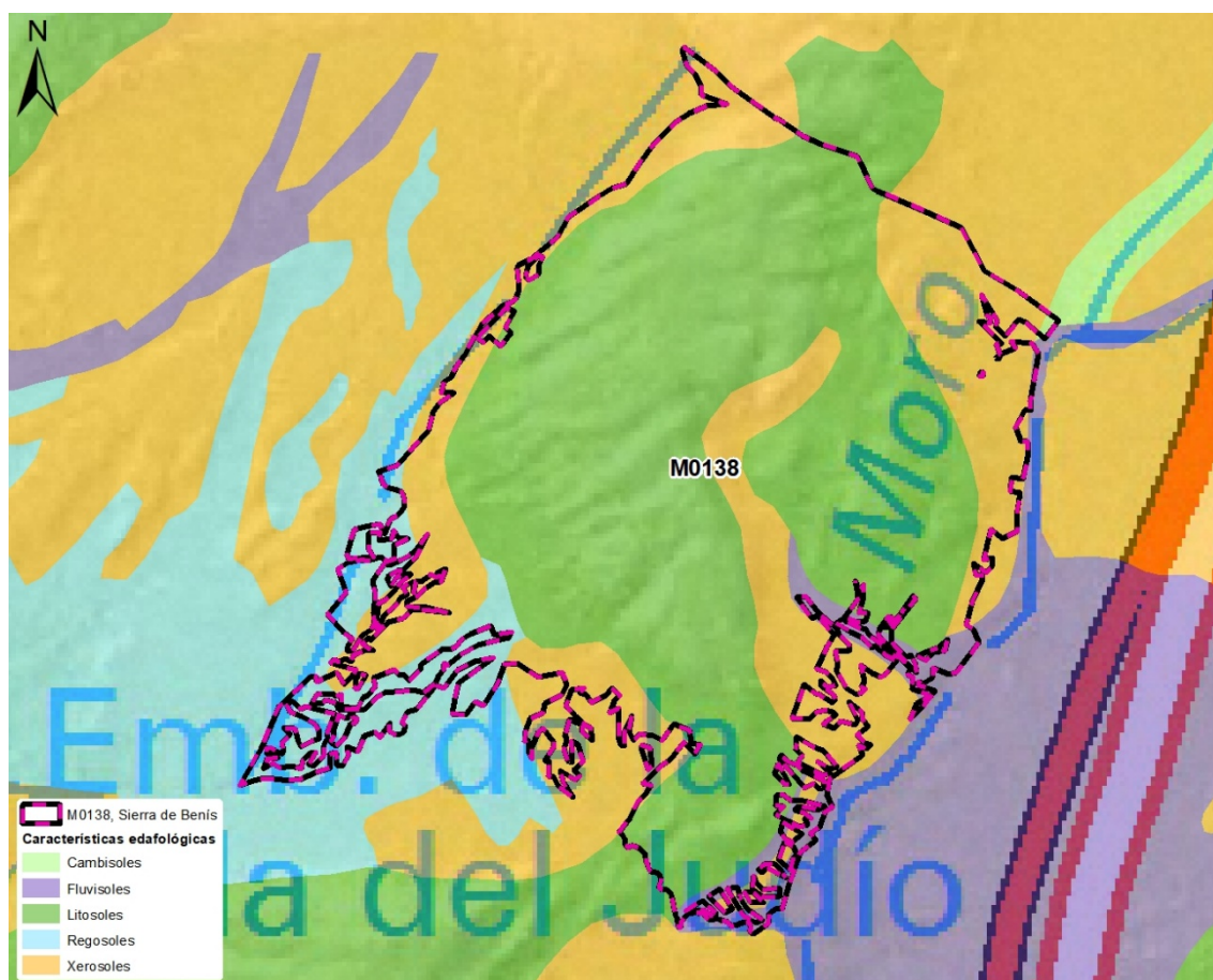
FIGURA 3. Características edafológicas
