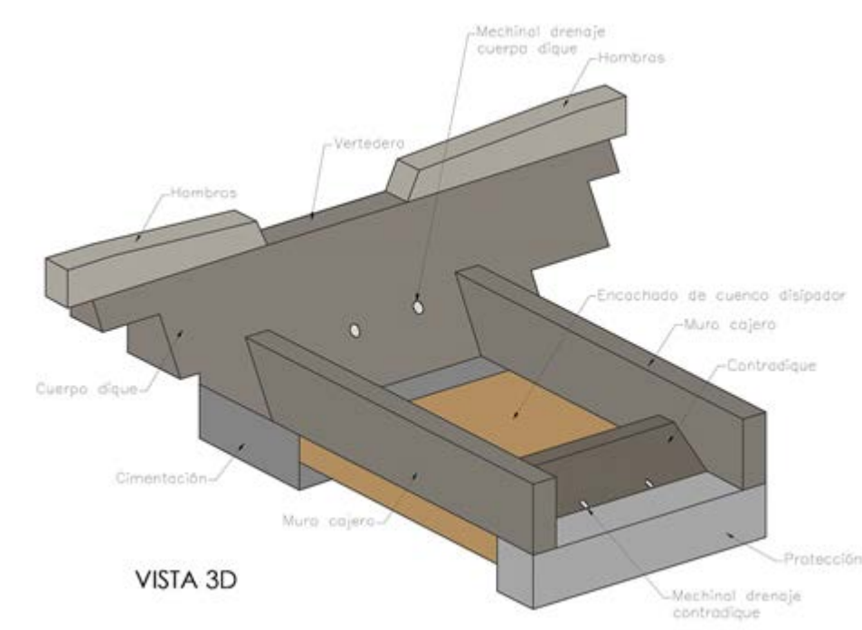
FIGURA 41. Modelo 3D de dique
