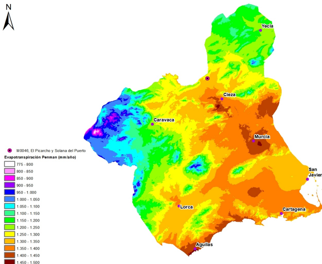
FIGURA 8. ETP
