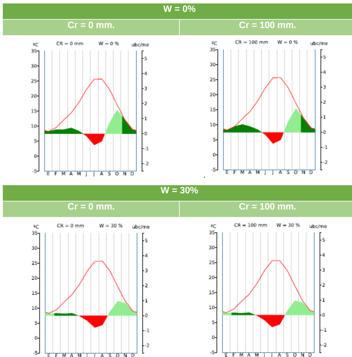
FIGURA 9. Diagramas bioclimáticos
