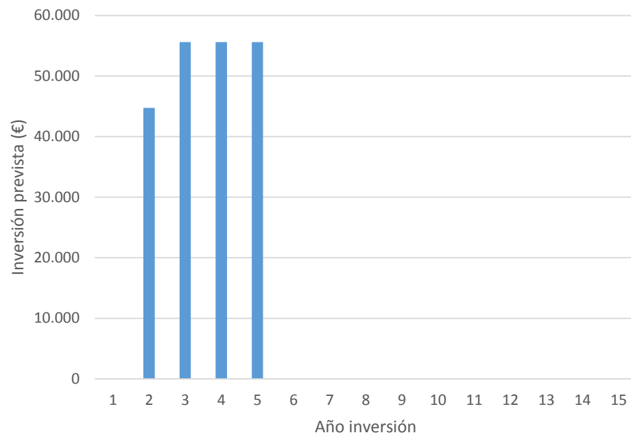
GRÁFICO 6. Inversión en actuaciones de restauración hidrológica por anualidades en los MUP – 48 y MUP – 149
