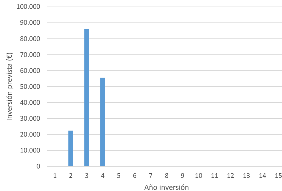
GRÁFICO 6. Inversión en actuaciones de restauración hidrológica por anualidades en los MUP – 48 y MUP – 149
