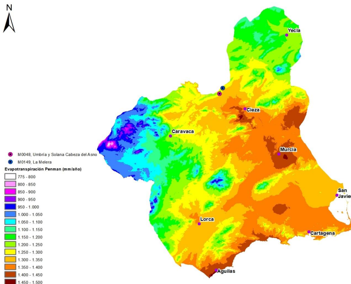
FIGURA 8. ETP
