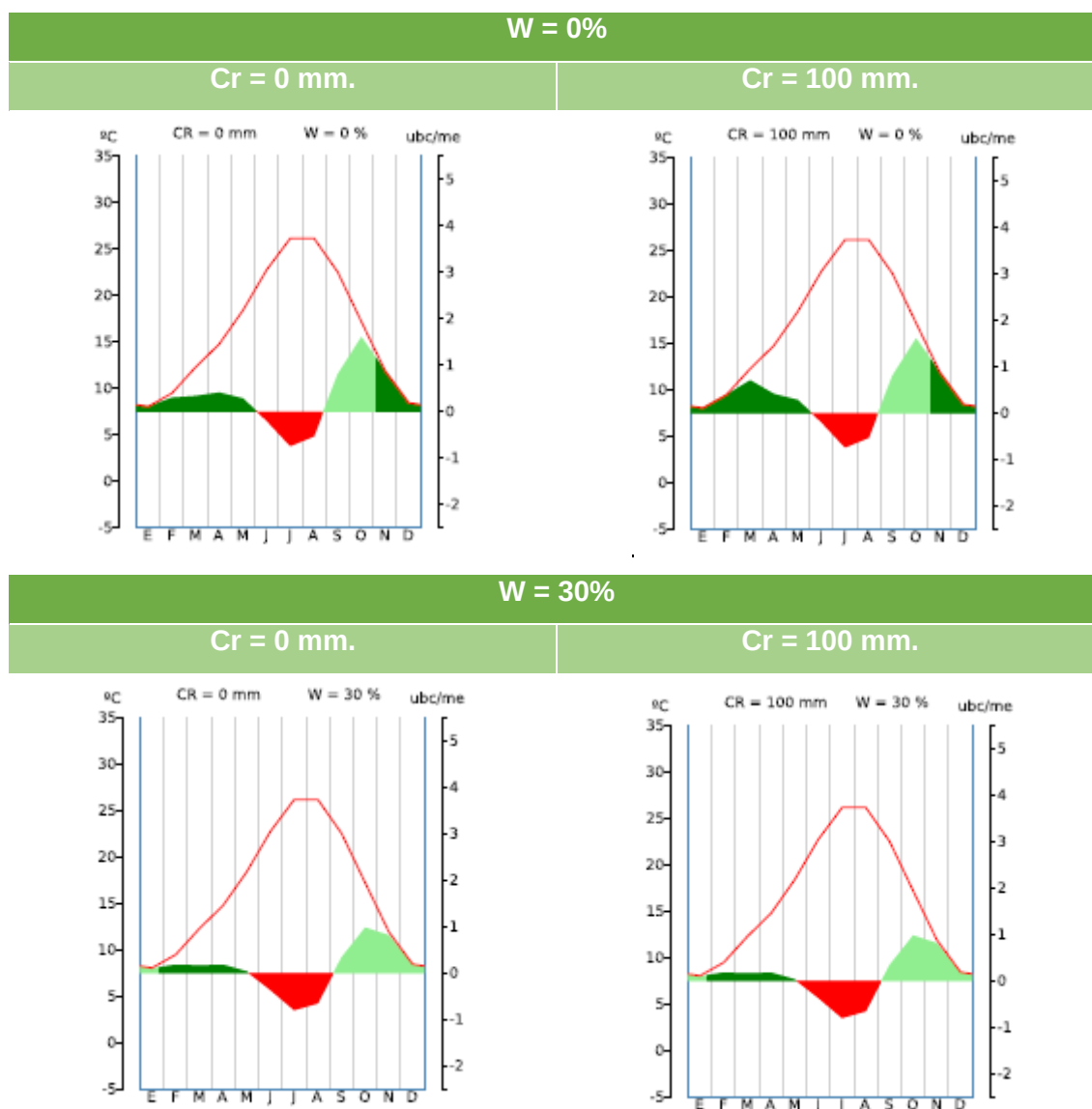
FIGURA 9. Diagramas bioclimáticos
