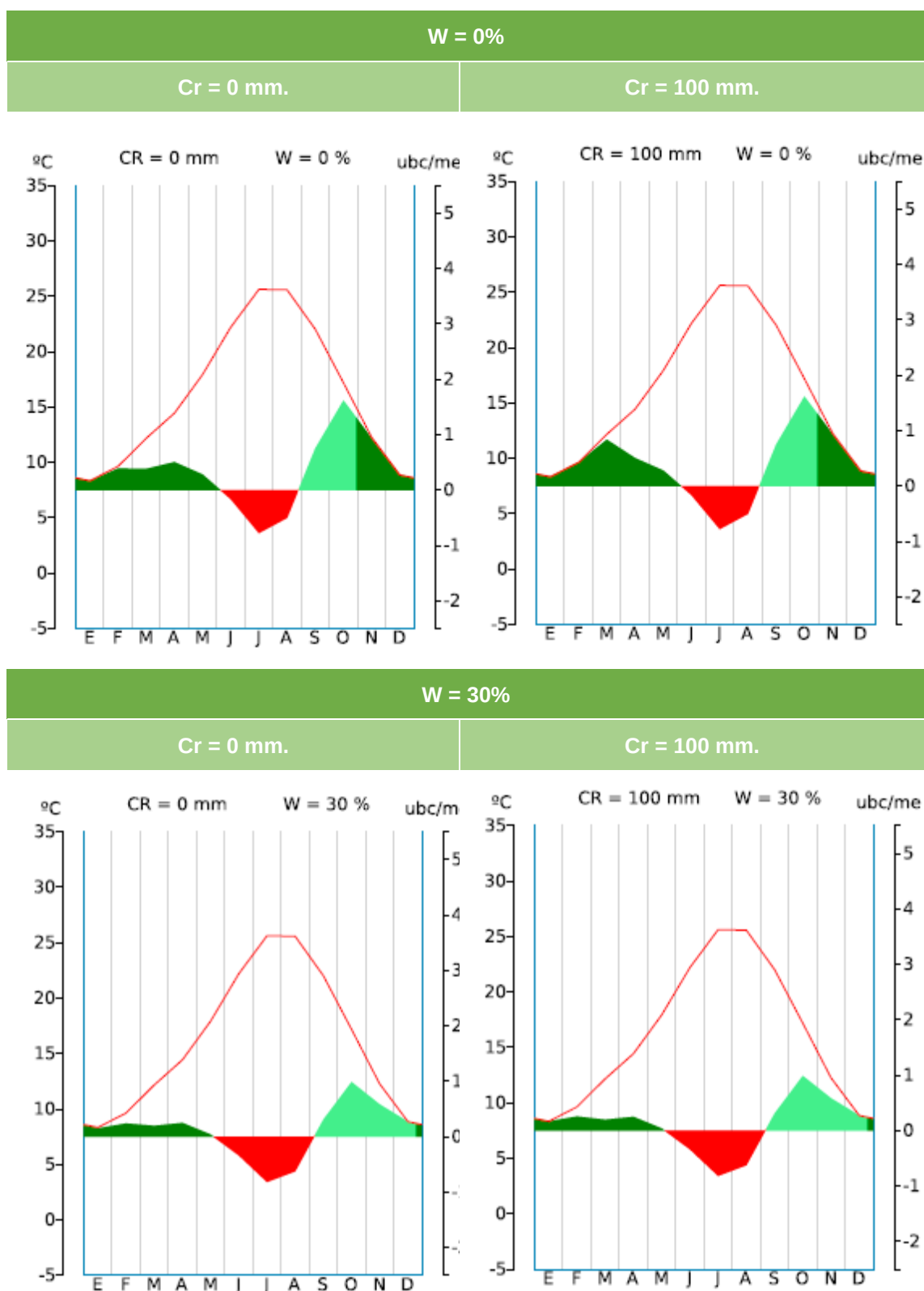
FIGURA 9. Diagramas bioclimáticos MUP – 142
