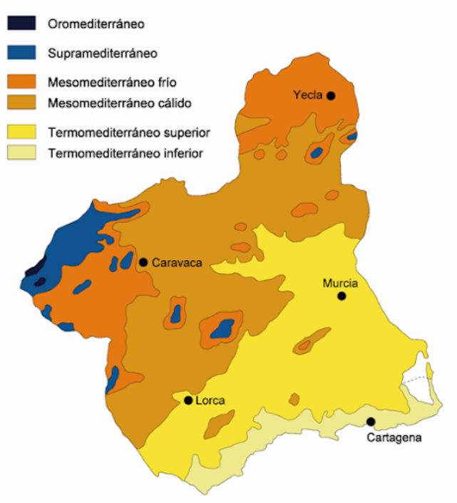
FIGURA 39. Termotipos para la región de Murcia
