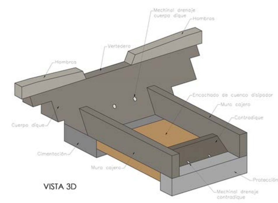
FIGURA 42. Modelo 3D de dique
