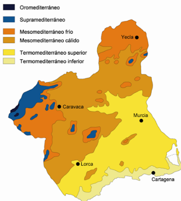
FIGURA 36. Termotipos para la región de Murcia
