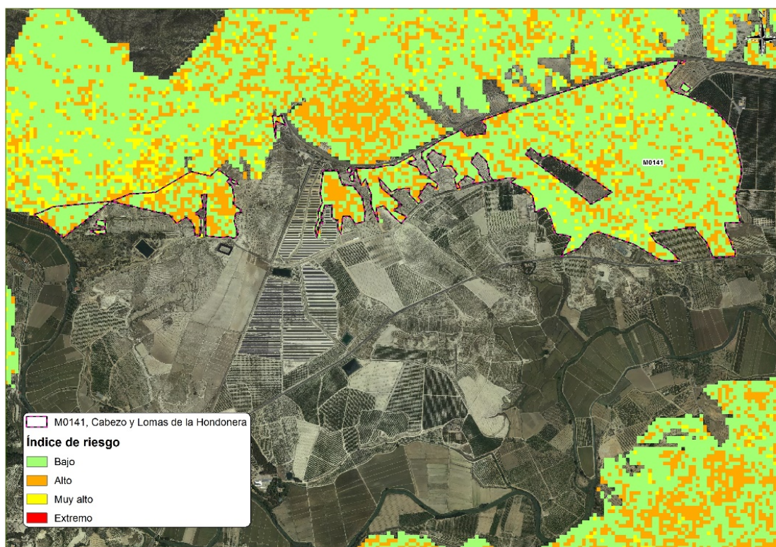
FIGURA 23. Riesgo de incendio
