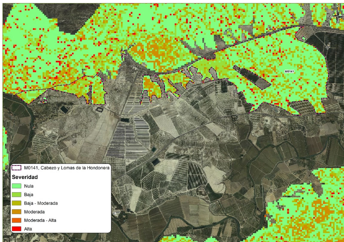
FIGURA 22. Severidad del incendio
