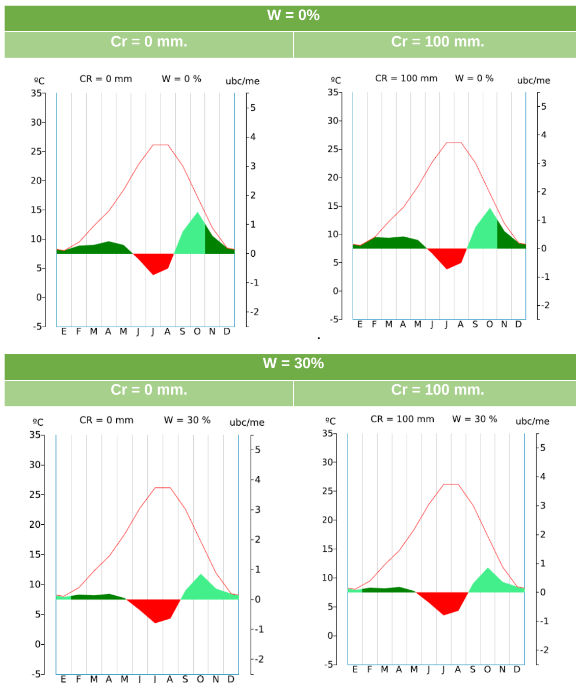
FIGURA 9. Diagramas bioclimáticos MUP – 141
